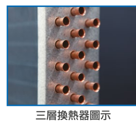
三層換熱器圖示
